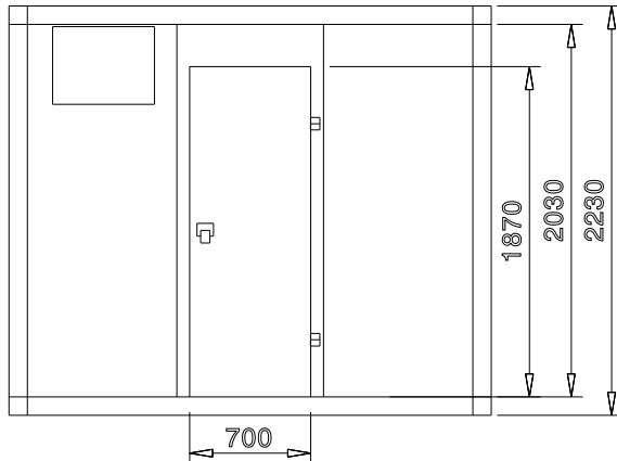
Front aanzicht
